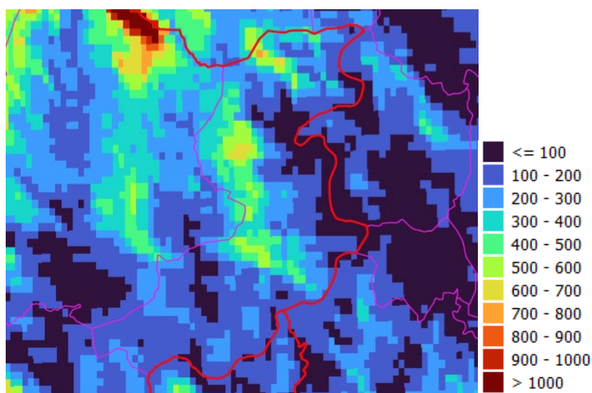
Figura 4. Densidade de potencia de vento media en Crecente (50m) [7]
