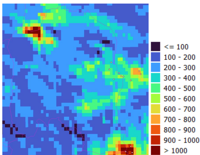
Figura 4. Densidade de potencia de vento media en Cuntis (50m) [7]
