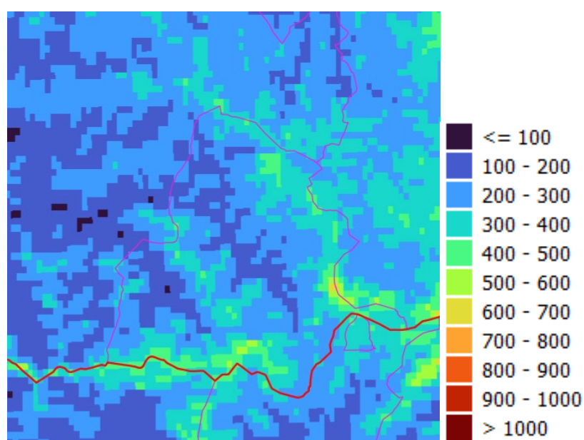
Figura 3. Densidade de potencia de vento media en Dozón (50m) [6]
