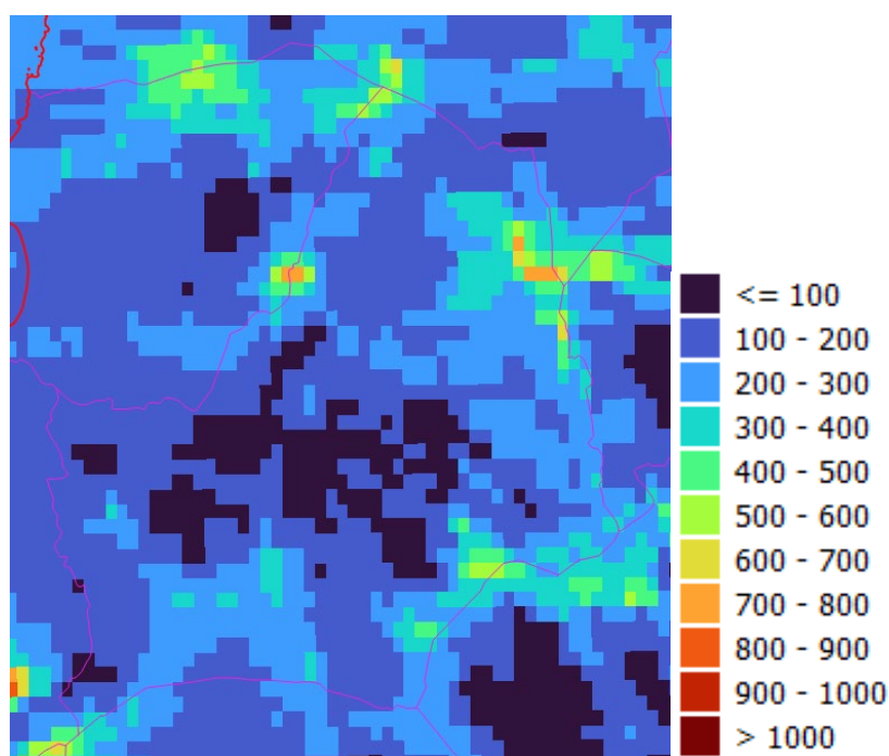
Figura 3. Densidade de potencia de vento media en Gondomar (50m) [6]
